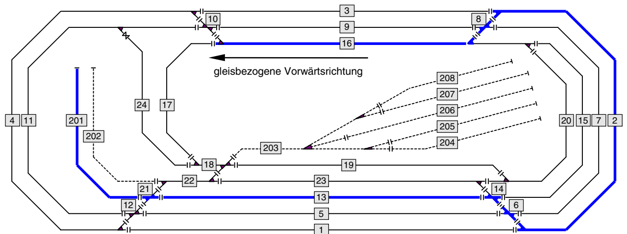
Bild 43.2 Verlauf der Route Nr. 2
