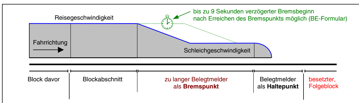
Bild 21.4a Geschwindigkeitsverlauf beim Bremsen mit Verzögerung
