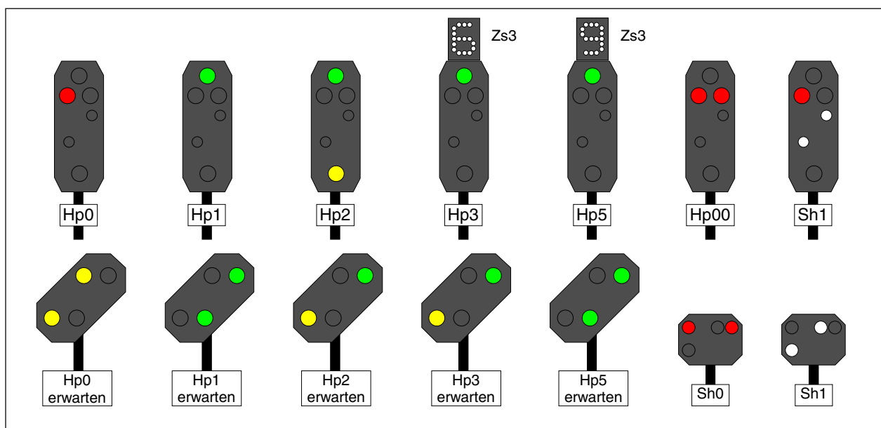
Abbildung 71: Signalbilder für Landeskennung D (DB Deutsche Bahn) und Zs3 > 40 km/h
