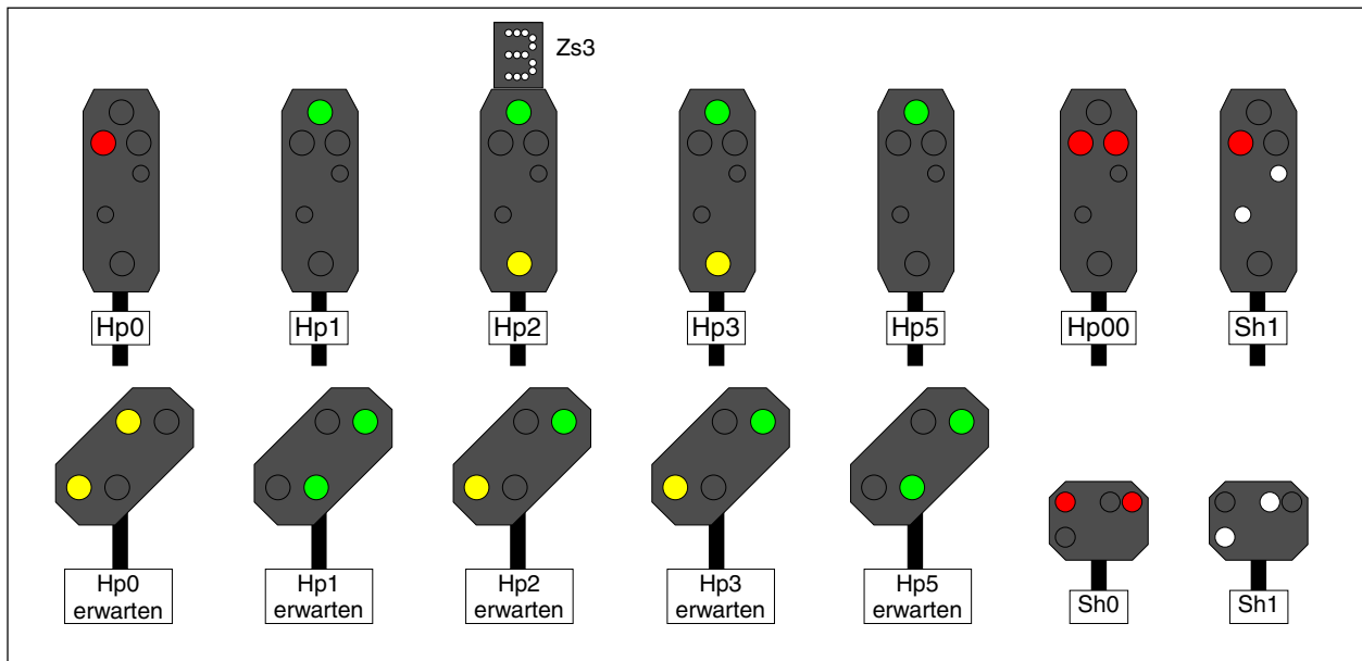
Abbildung 72: Signalbilder für Landeskennung D (DB Deutsche Bahn) und Zs3 < 40 km/h
