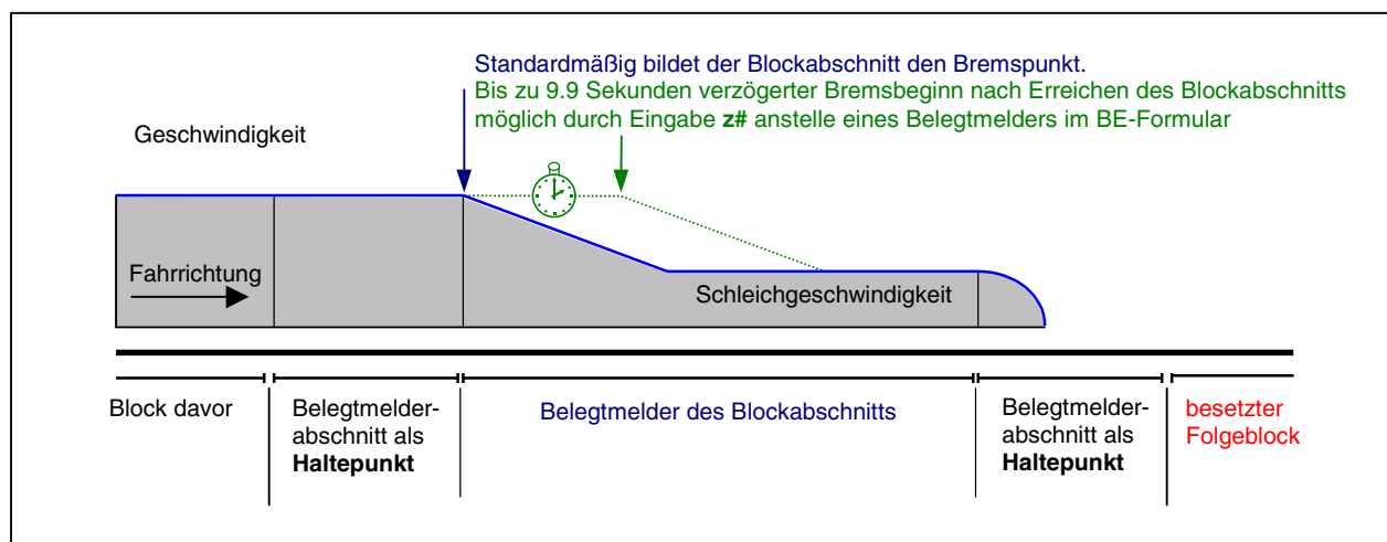
Bild 21.5 Ohne Bremspunkt beginnt das Bremsen am Blockabschnitt
