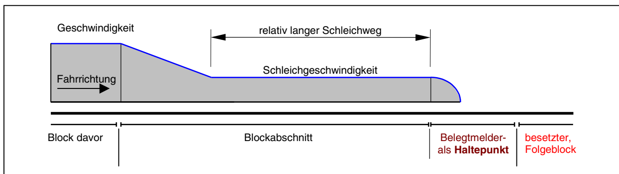
Bild 21.3 Geschwindigkeitsverlauf bei Anordnung eines Haltepunkts
