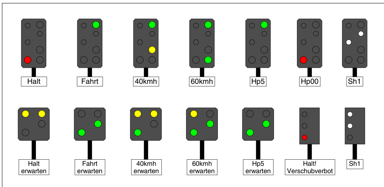
Abbildung 73: Signalbilder für Landeskennungen A und O (ÖBB Österreich)
