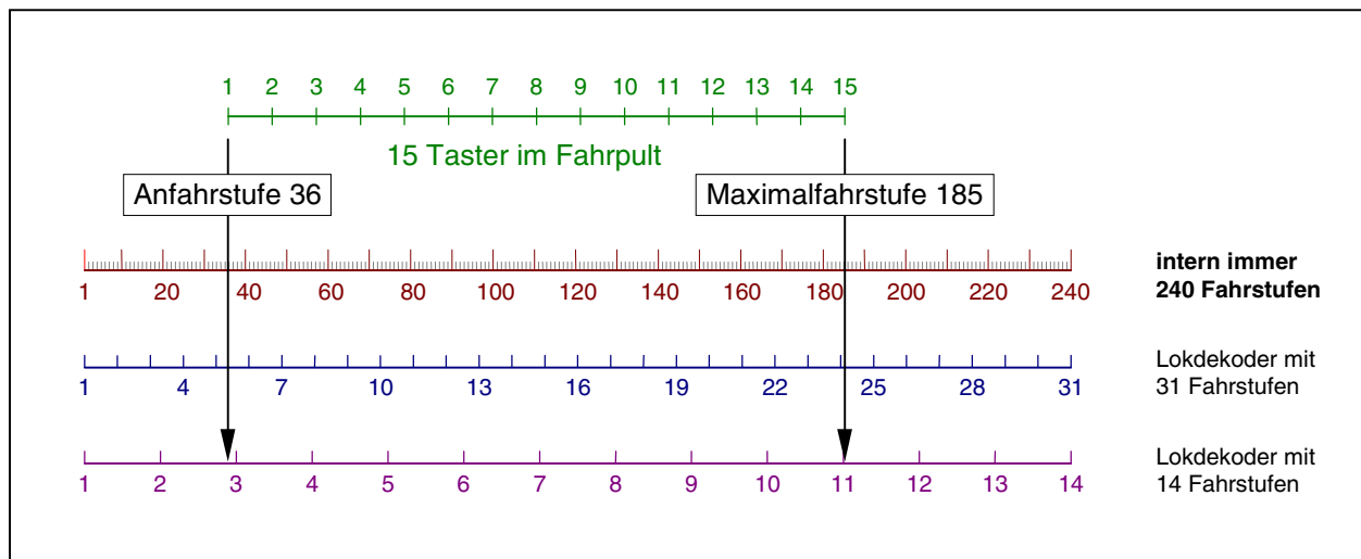
Abbildung 57: Fahrpultstufen und Geschwindigkeitsstufen
