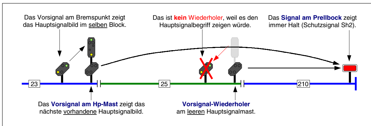
Abbildung 70: Landeskennung D: Das Vorsignal für ein Sh2-Schutzsignal am Prellbock ist dunkel.
