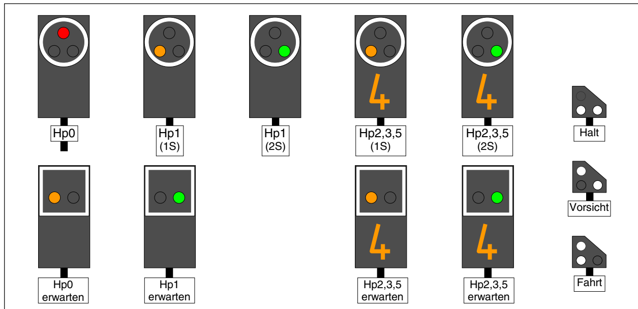
Abbildung 76: Signalbilder für Landeskennung C (SBB Schweiz, 'System N')
