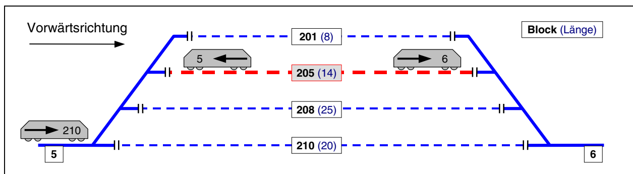
Bild 41.1: Ausfahr- und Ausweichautomatik in einem 4-gleisigen Schattenbahnhof
