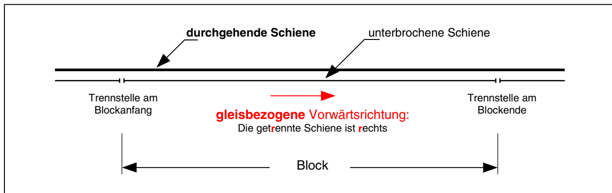
Bild 21.1 Prinzipskizze: Grundmerkmale eines Blocks
