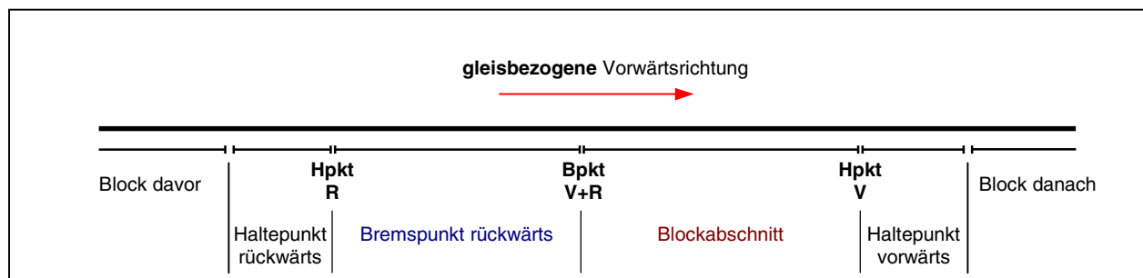
Bild 21.6 Zwei Haltepunkte und ein einseitiger Bremspunkt
