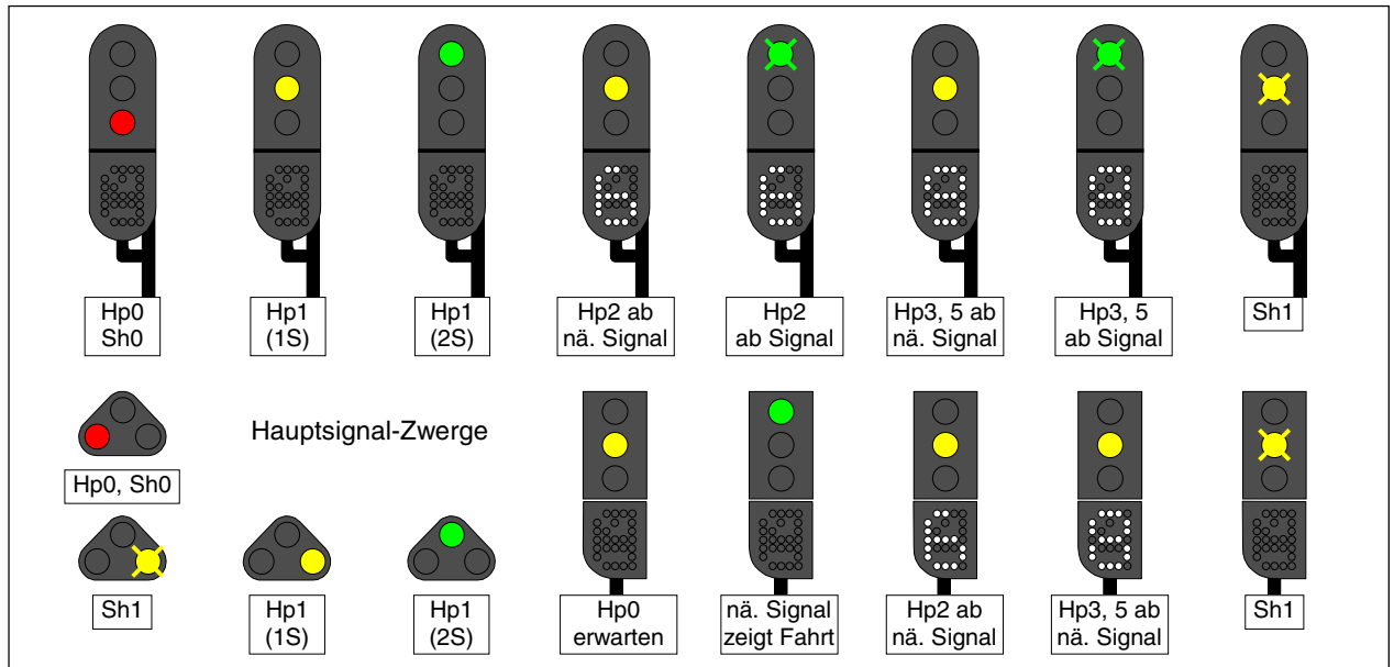
Abbildung 78: Signalbilder für Landeskenntung N (NS Niederlande)
