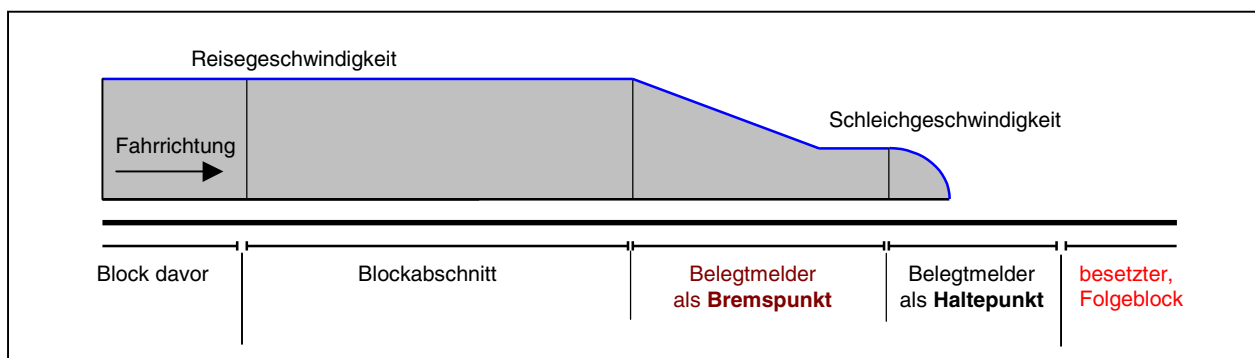
Bild 21.4 Geschwindigkeitsverlauf bei Anordnung eines Bremspunkts und eines Haltepunkts
