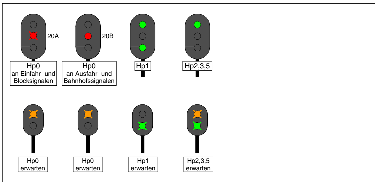
Abbildung 75: Signalbilder für Landeskenntung R (NSB Norwegen)
