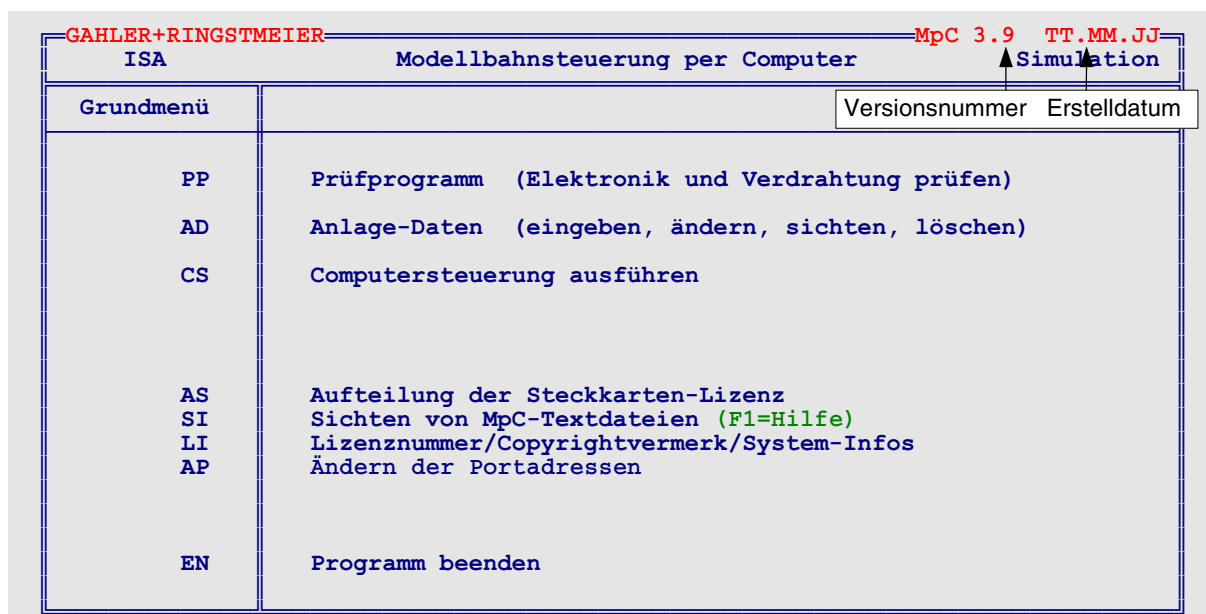
Abbildung 3: Bildschirm des Grundmenüs (MpC-Classic)
