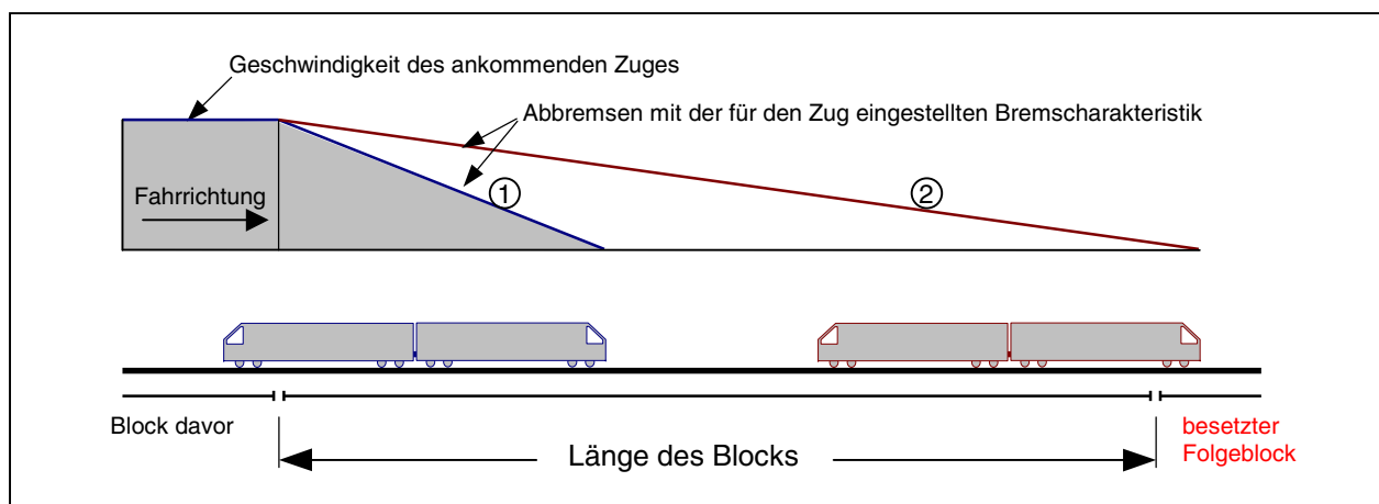
Bild 21.2 Beispiel für zu niedrige (1) und zu hohe (2) Bremscharakteristik
