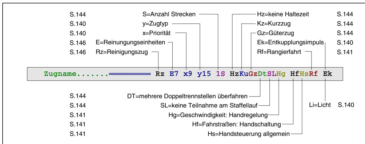
Abbildung 60: Bedeutung der unteren Zeile der Fahrregler-Anzeigen (MpC-Classic)
