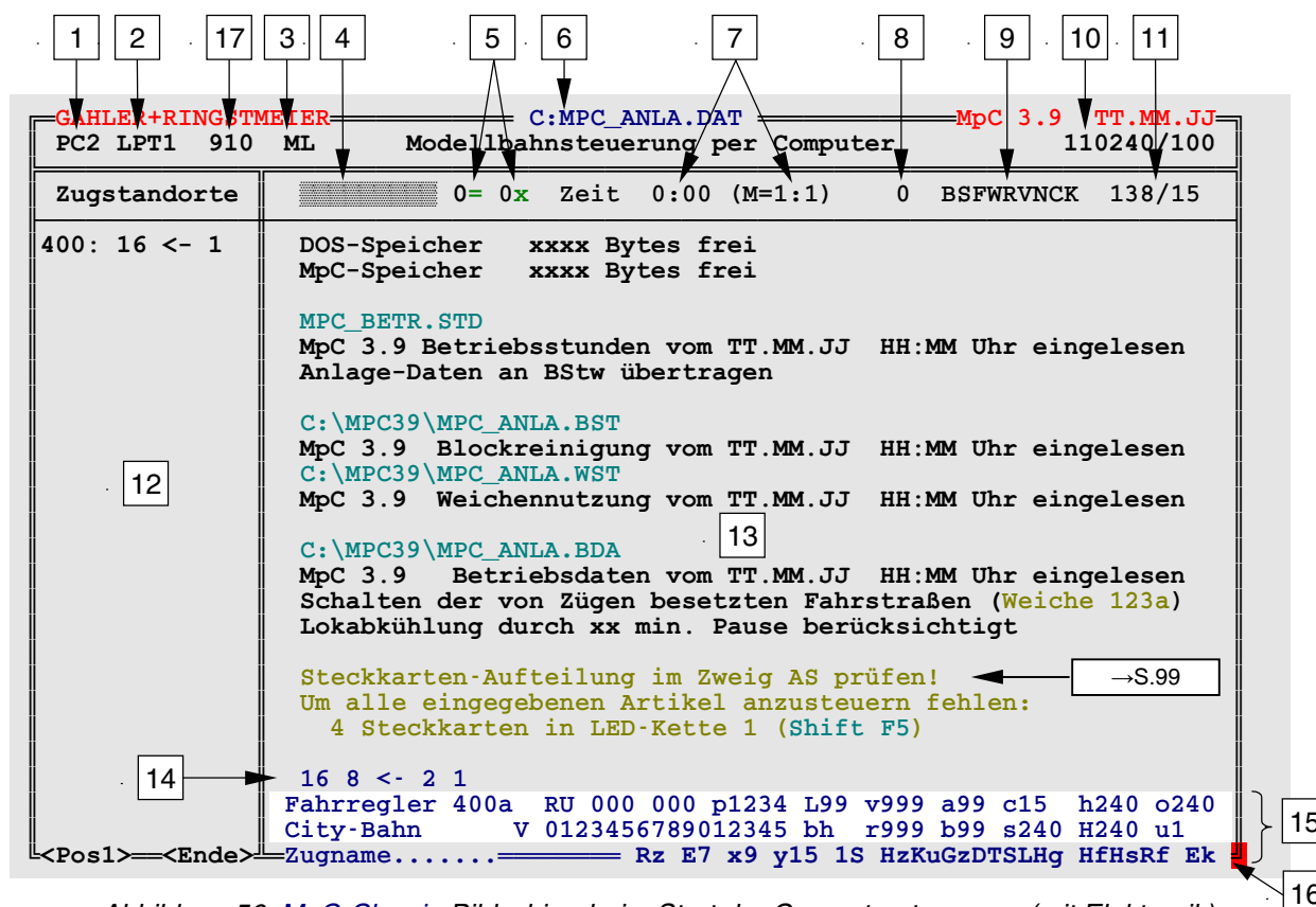
Abbildung 56: MpC-Classic-Bildschirm beim Start der Computersteuerung (mit Elektronik)
