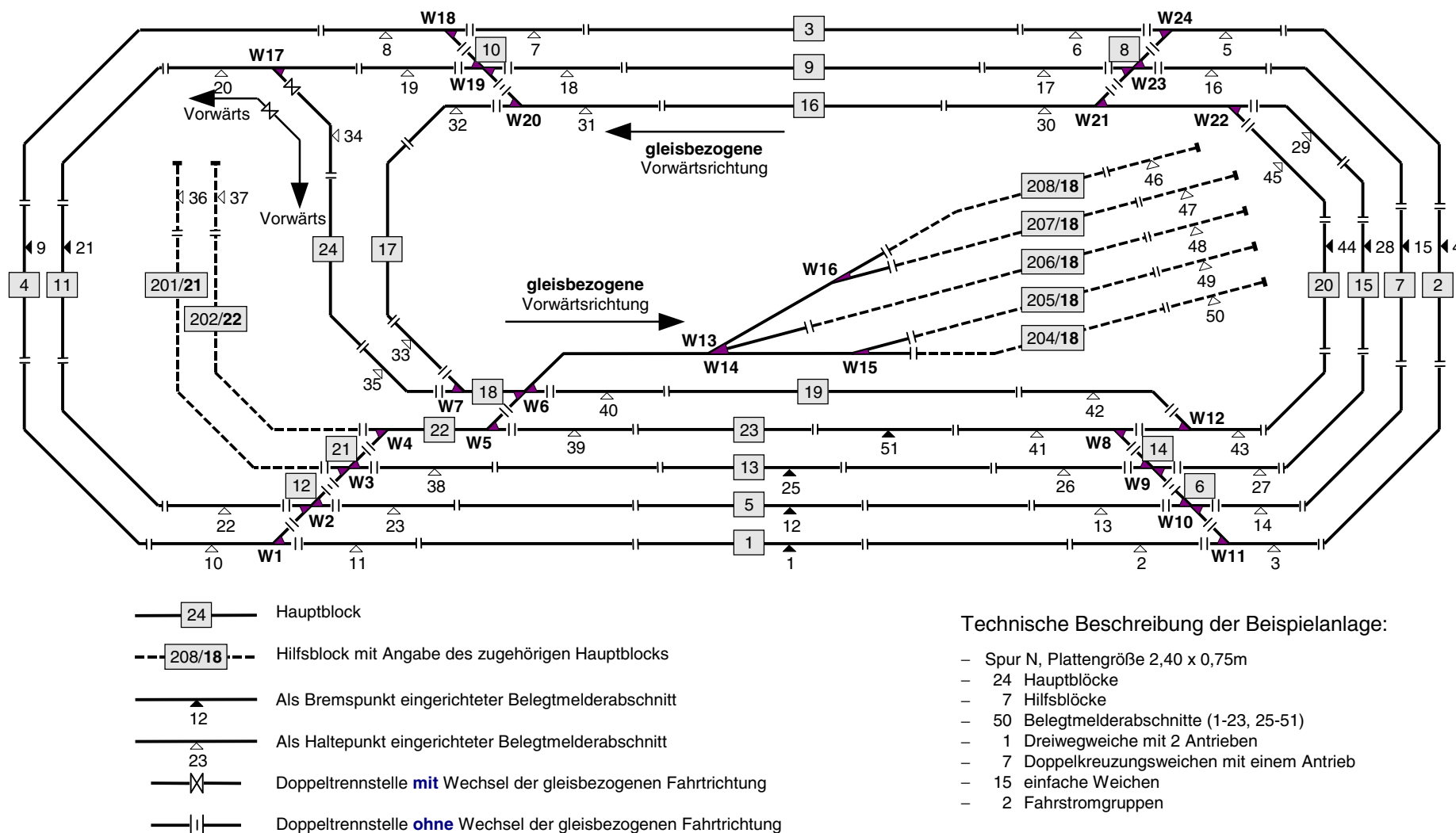
Bild 25.1a Anordnung der Halte- und Bremspunkte in der Beispielanlage (MPC-Classic)
