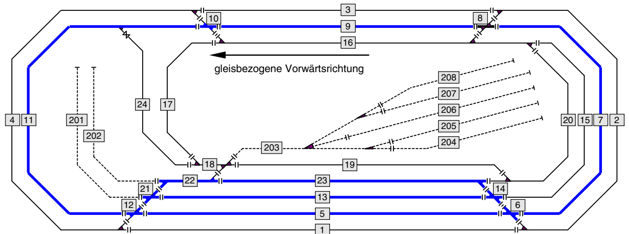
Bild 43.1 Verlauf der Route Nr. 1
