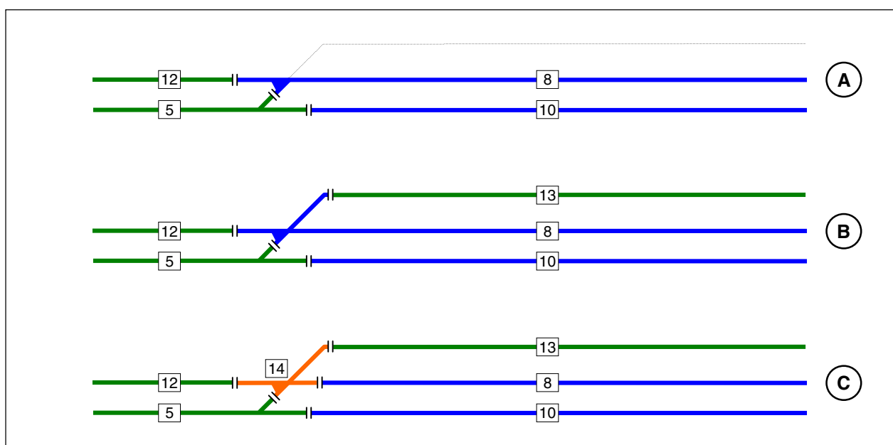
Bild 23.2 Eine Doppelkreuzungsweiche wird zu einem einzelnen Block
