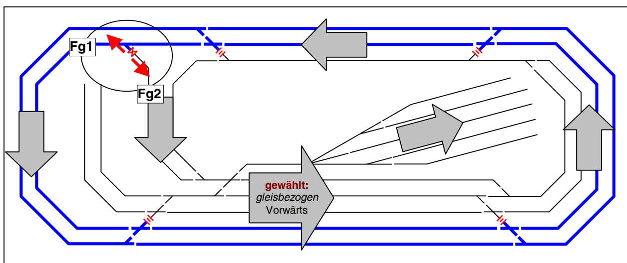
Abbildung 79: Wahl der gleisbezogenen Vorwärtsrichtung und Festlegen der Doppeltrennstellen
