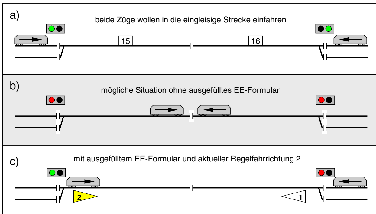
Abbildung 34: Eine aus den Blöcken 15 und 16 bestehende eingleisige Strecke
