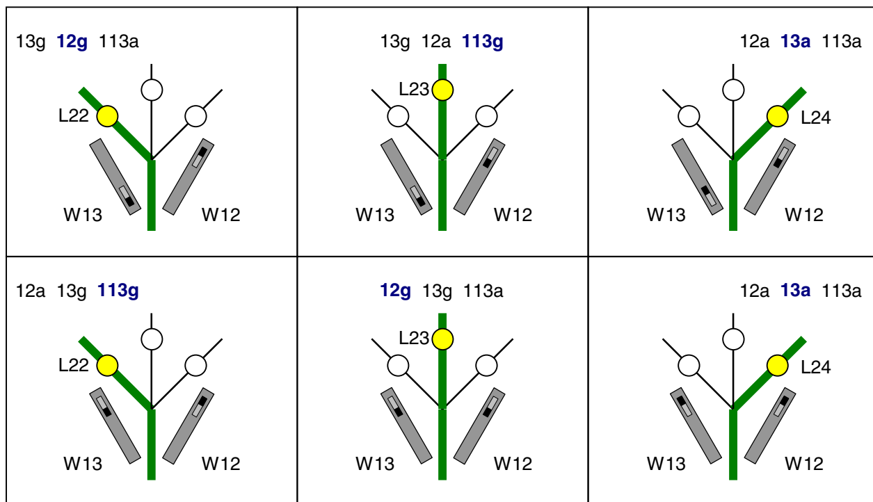
Bild 12.5 Schaltreihenfolge der beiden Antriebe einer Fleischmann-Piccolo-Dreiwegweiche Die drei Stells-LED sind jeweils den fettgedruckten Weichenlagen zugeordnet
