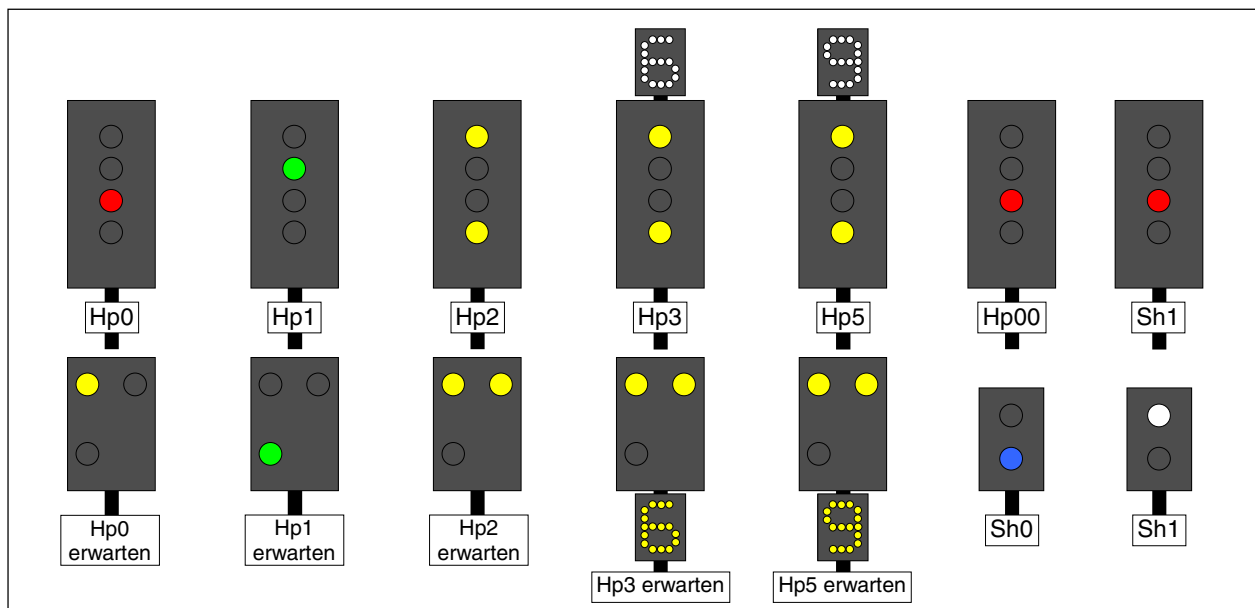
Abbildung 74: Signalbilder für die Landeskenntung L (CFL Luxemburg)
