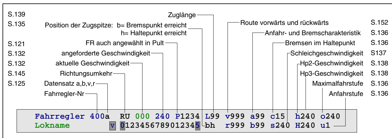
Abbildung 59: Bedeutung der Fahrregler-Anzeigen (MpC-Classic und MpC-Digital)
